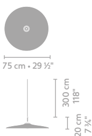
pendant light
